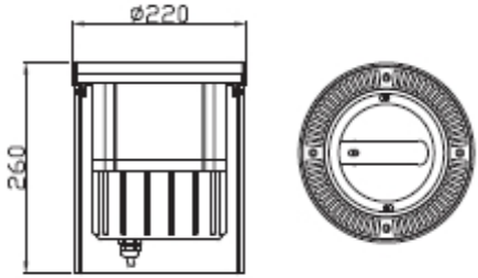
A: 一体式尺寸图
