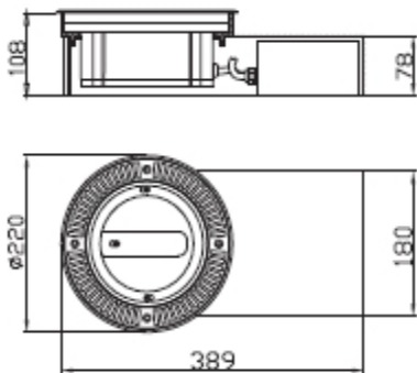
B: 分体式尺寸图
